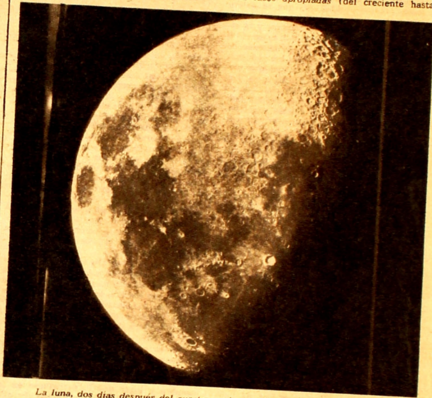
La luna, dos días después del cuarto creciente. (Fot. Observatorio Yerkes).
