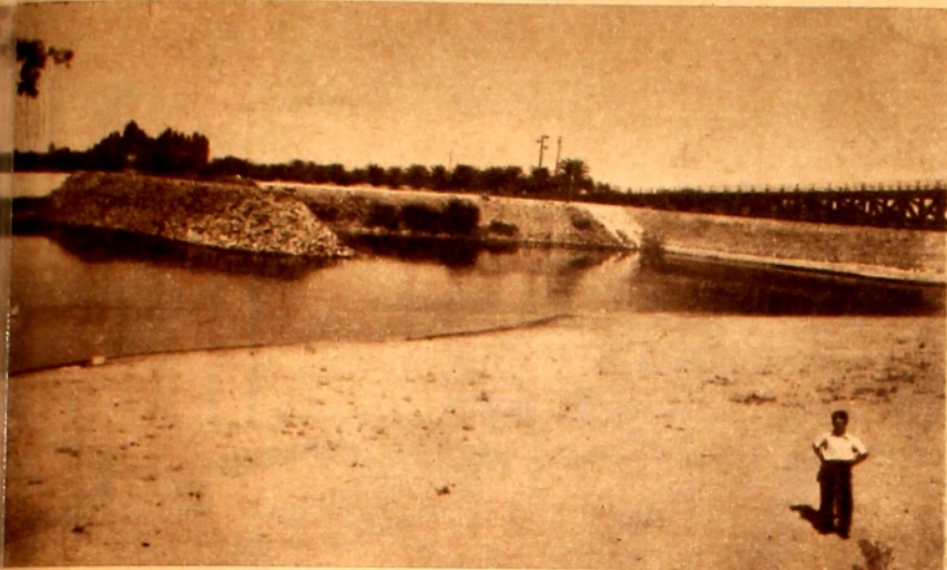
Espigones de piedra dispuestos para rectificar al río Santa Lucía que amenazaba con contornear el puente de Paso Pache, cortando las comunicaciones interdepartamentales.
