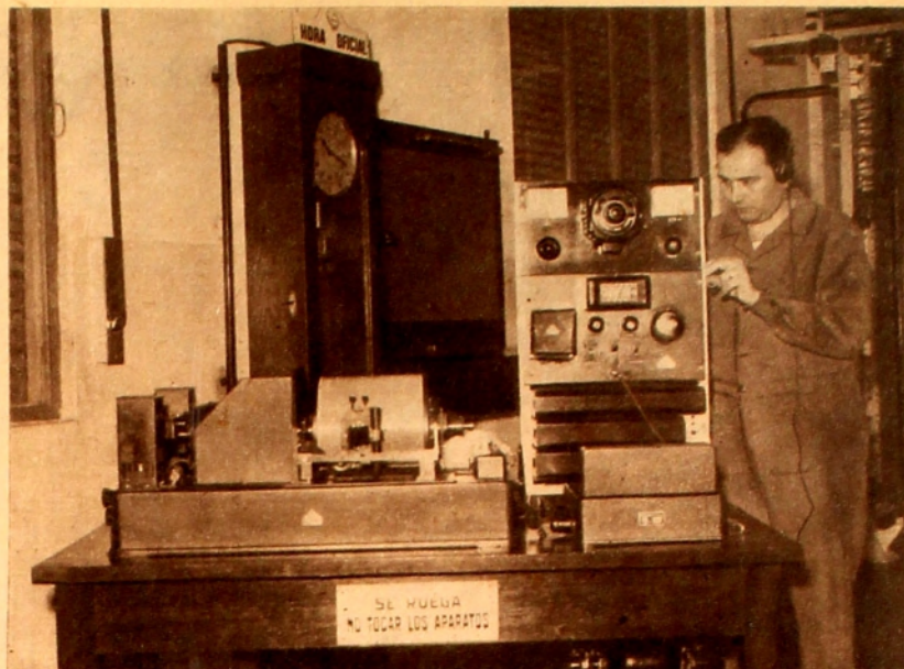
Las instalaciones de la "Hora Parlante", con el rodillo de las grabaciones y el trasmisor. Al fondo, conectada con los aparatos, la Hora Oficial, controlada diariamente por el Servicio Meteorológico.
