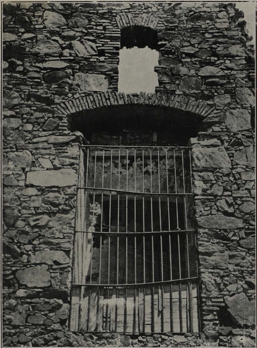
Fig. 54. — Muro del convento de San Francisco, dispuesto en “opus incertum” con ladrillos intercalados y la construcción de los arcos en ladrillo.
