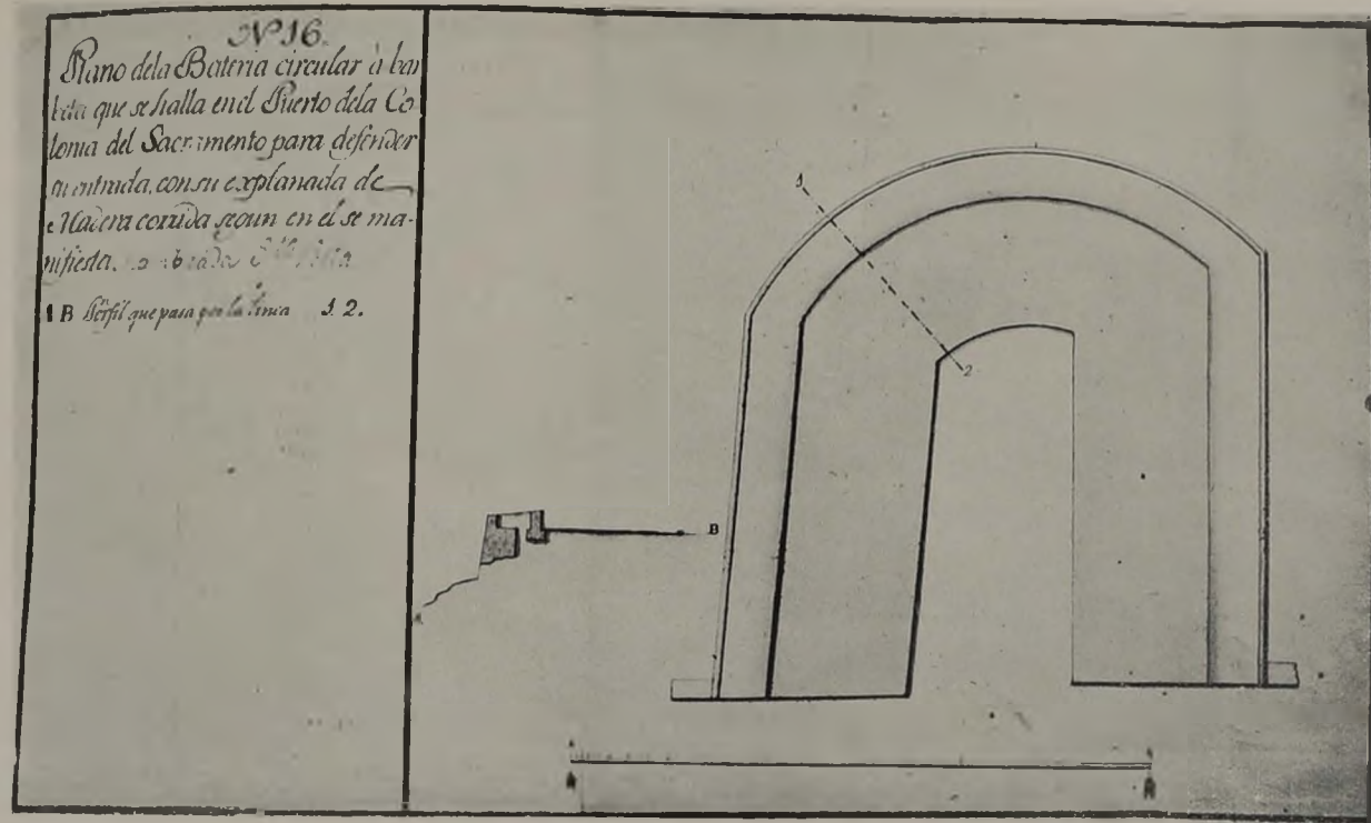
Fig. 38. — Plano de la Bateria de Santa Rita. — N.º del ejemplar, 16. N.º del plano, 116. Archivo del Cuerpo Español de Ingenieros, 1771-1808
