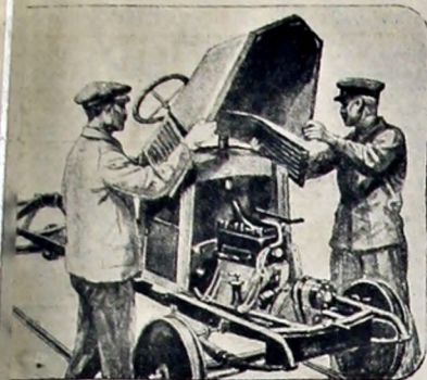
8. Después del radiador se procede a montar el capot o espaldón, el que se mantiene abierto mediante un especial dispositivo
