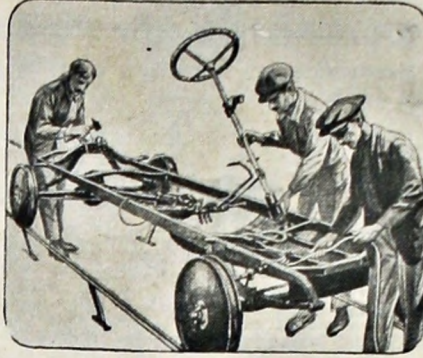
2. Mientras que un operario coloca las abrazaderas del elástico posterior, otro arma la dirección y un tercero fija los cables eléctricos.
