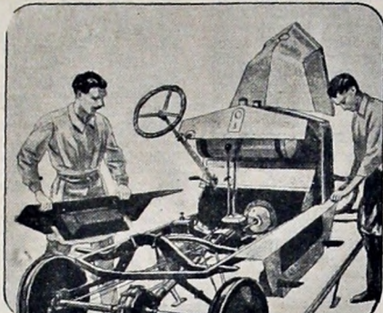
12. Sobre los largueros del chasis, se montan los cajones destinados a recibir la batería y las herramientas
