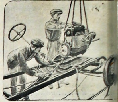
3. El motor ya armado (menos el magneto) ciende sobre el chasis, donde es fijado por cuatro bulones.—Otro operario arma el desembrague.
