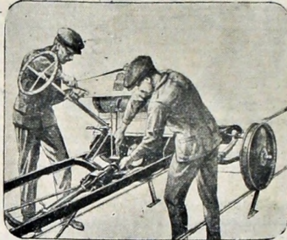
5. La barra de la dirección se fija al tablero, mientras que un compañero arma las palancas del cambio y del freno.
