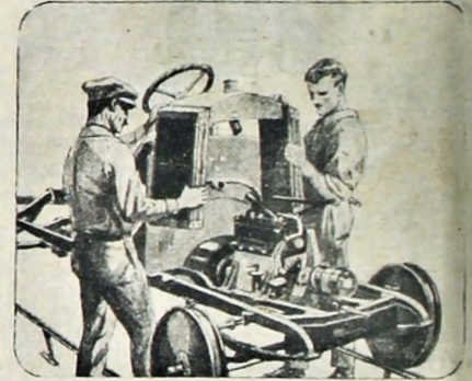
7. El radiador, compuesto de dos elementos de los verticales, con un colector central, se coloca en continuación, fijándolo fuertemente al chasis.
